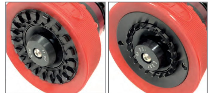
Gefräste Aluminiumzähne
